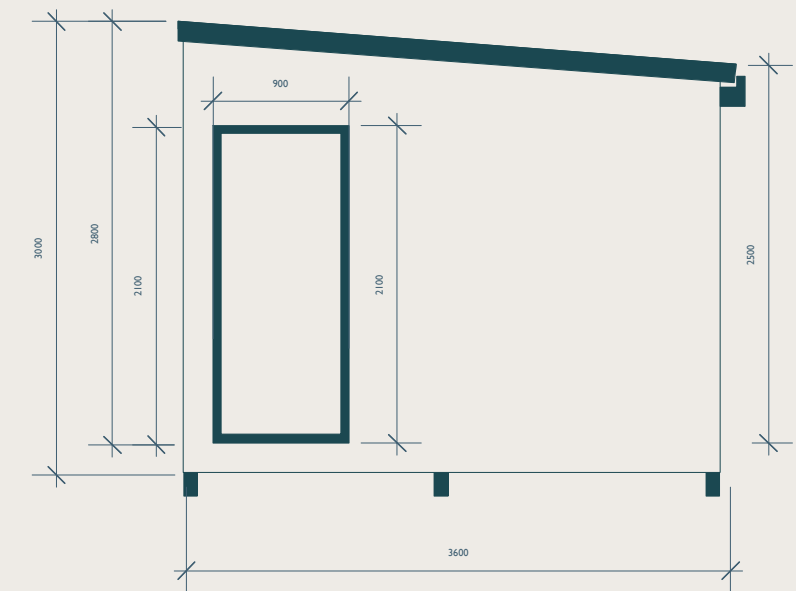
Right Elevation
