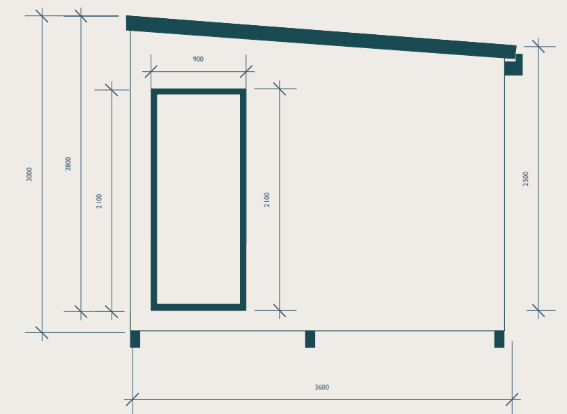
Right Elevation
