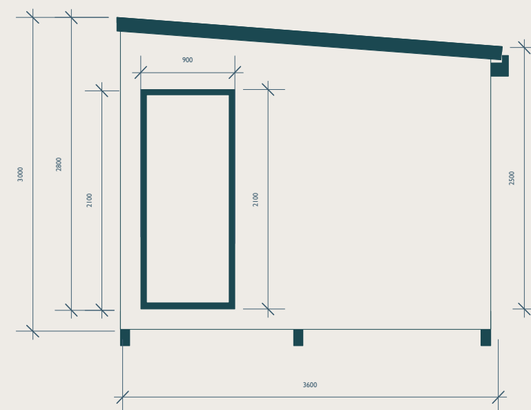
Right Elevation
