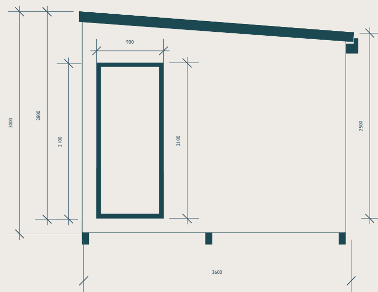
Right Elevation
