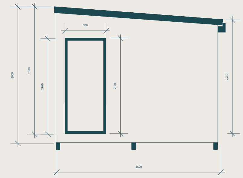
Right Elevation
